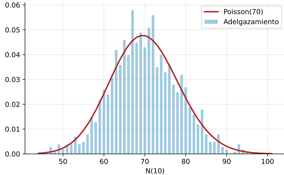
N(10) en 1000 corridas
